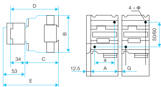
CD1 9 - CD4 32
