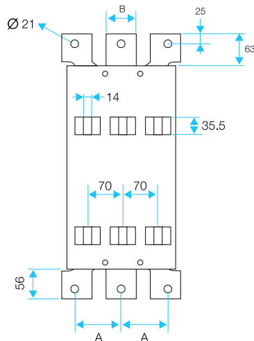
1250A - 1600A
