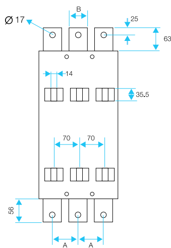
1000A
