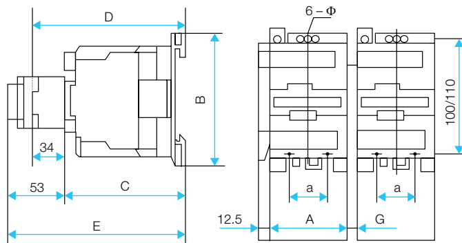
CD5 40 - CD6 95
